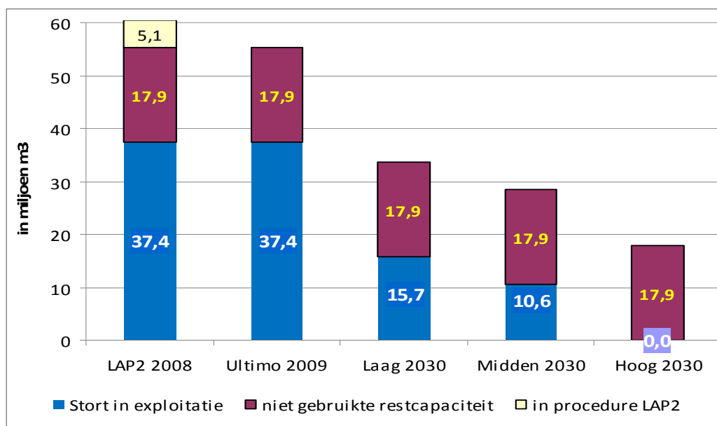
Figuur 6: Restcapaciteit volgens uitgangssituatie en per scenario (in Mm 3 )
